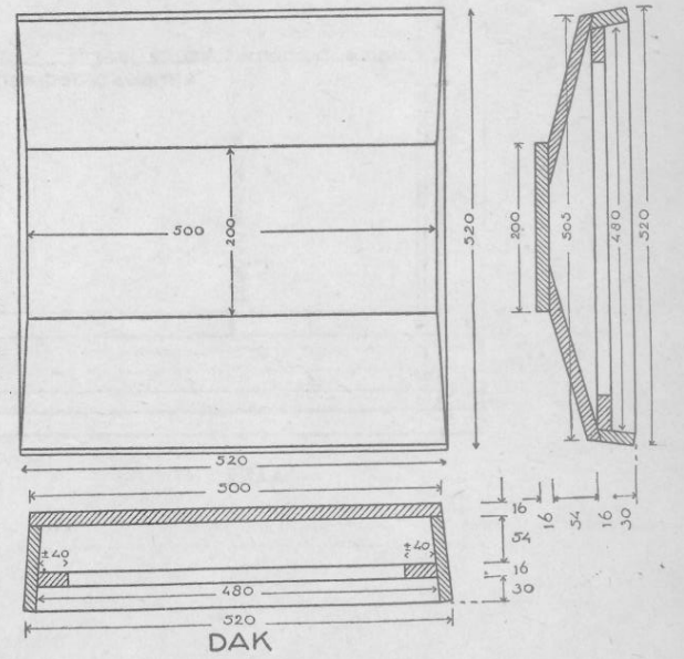
DAK
