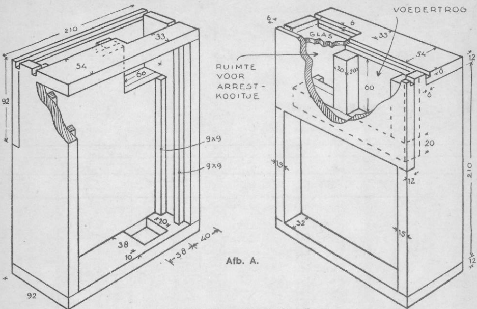
BEVR. KASTJE
