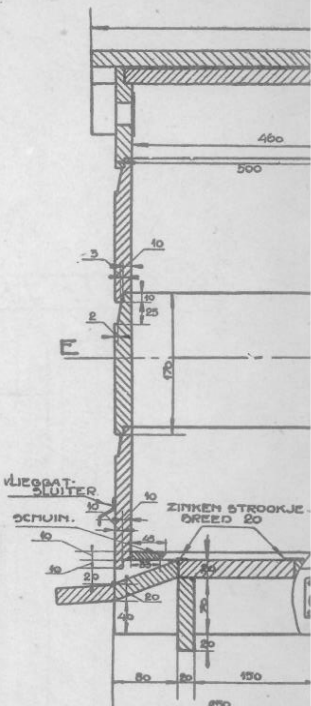
DOORSNEDE A-B.
