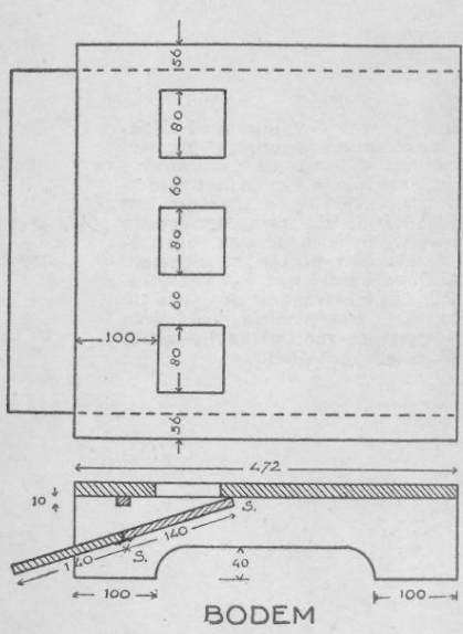
BODEM
