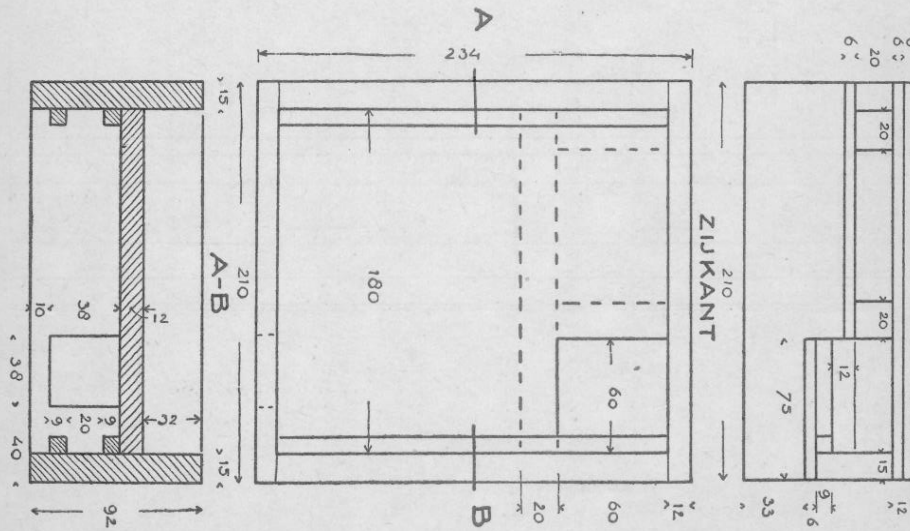
BEVR. KASTJE
